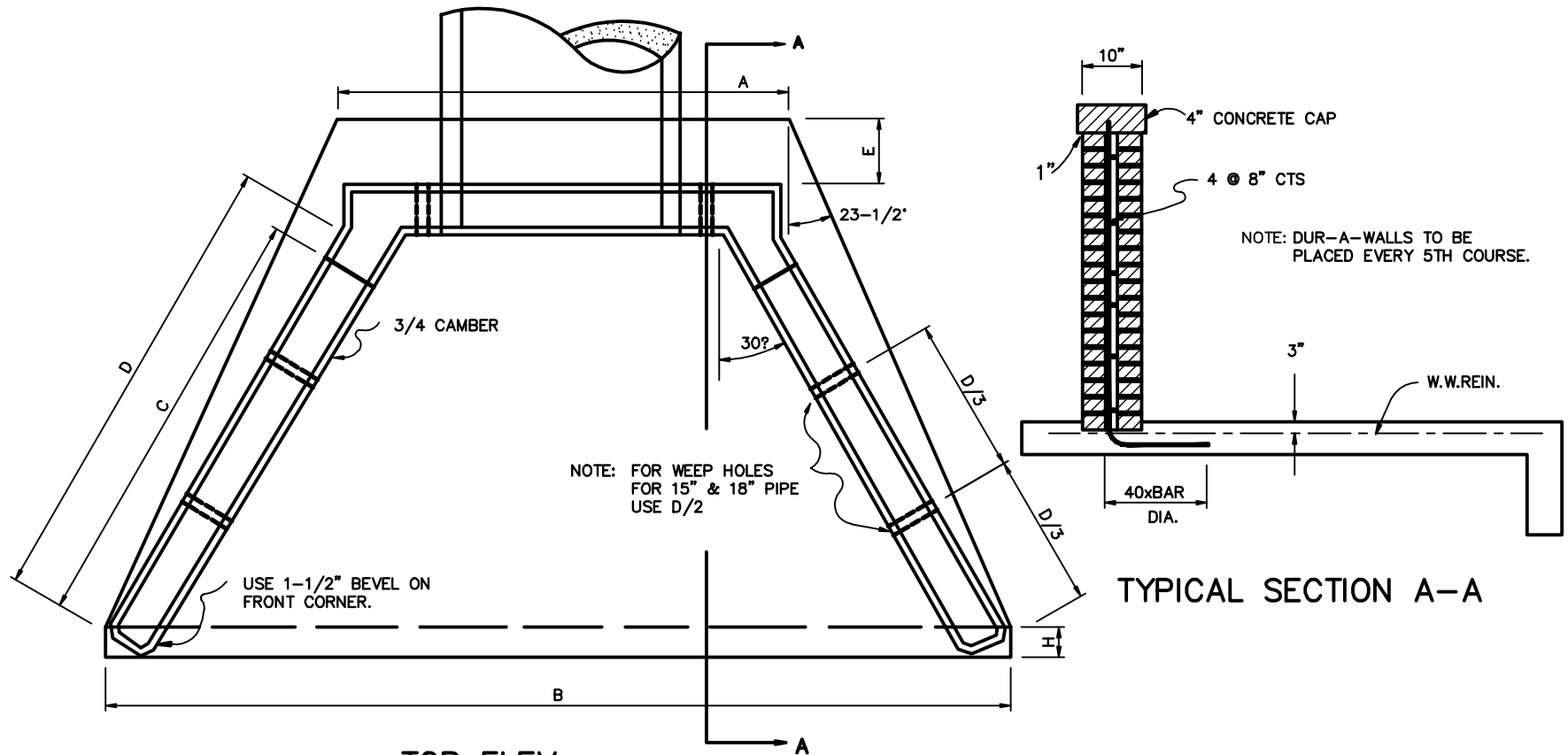
TOP ELEV.
