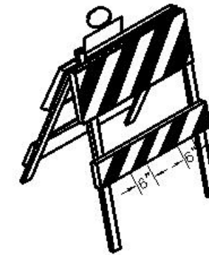
TYPE II BARRICADE
