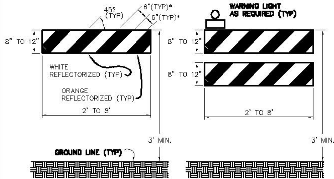
TYPE I BARRICADE
